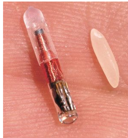
BILD: RFID-Chip-Implantat im Größenvergleich mit einem Reiskorn
